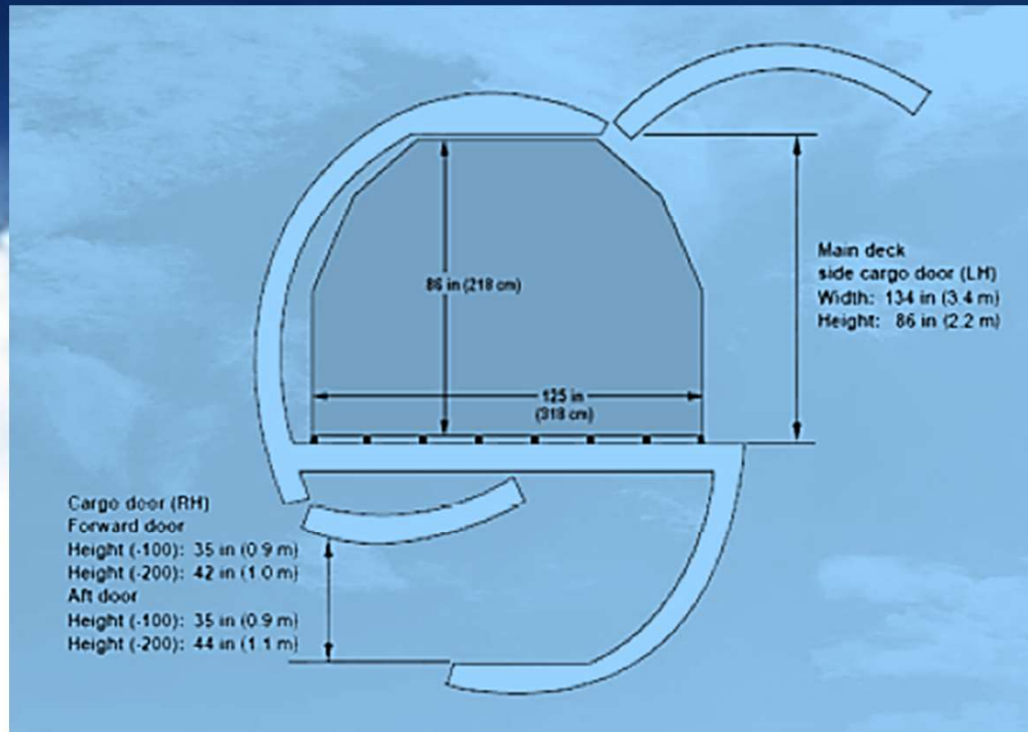
Dimensões das Portas de Carga
